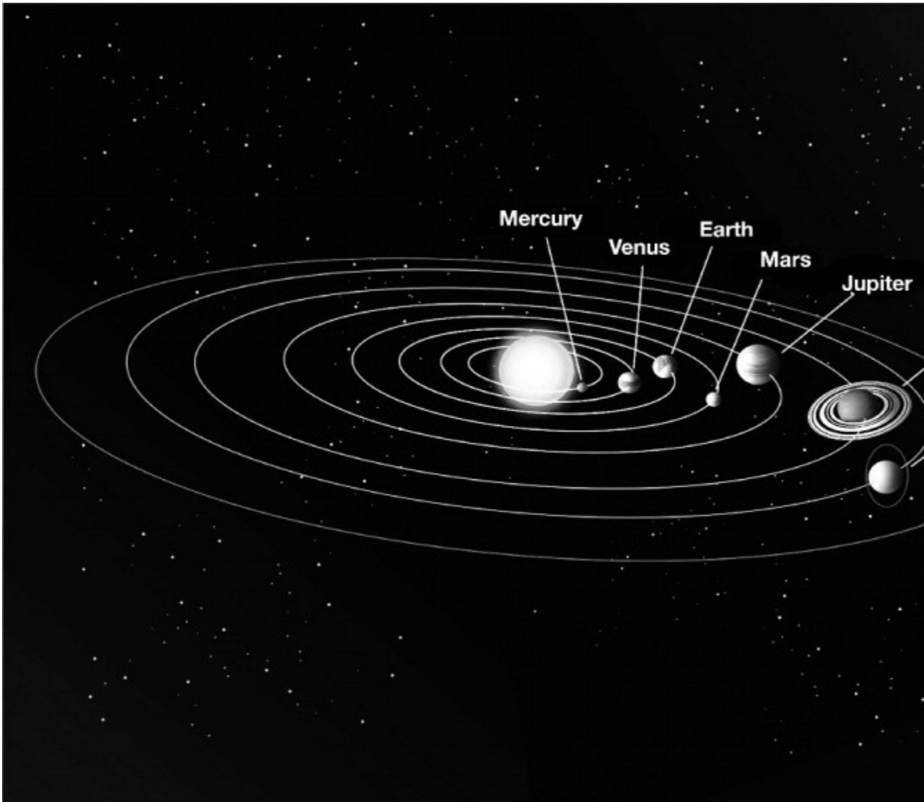
Abbildung 10 – Planetensystem
